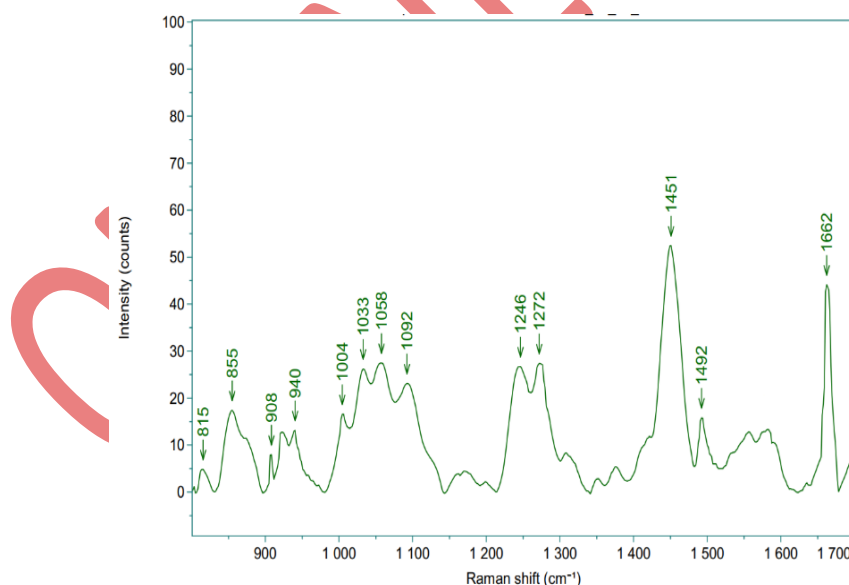
Hình 5. Phổ Raman trung bình chân bì của 10 mẫu mô da tươi được cố định formalin
